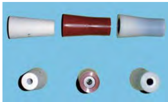
一般ノズル セラミック(左) ボロンSOFT(中) ボロンHARD(右)
